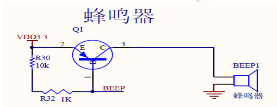
图一 蜂鸣器原理图
