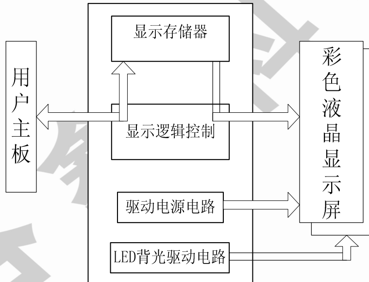
图 1 TFT6448BS-5.7 原理框图
